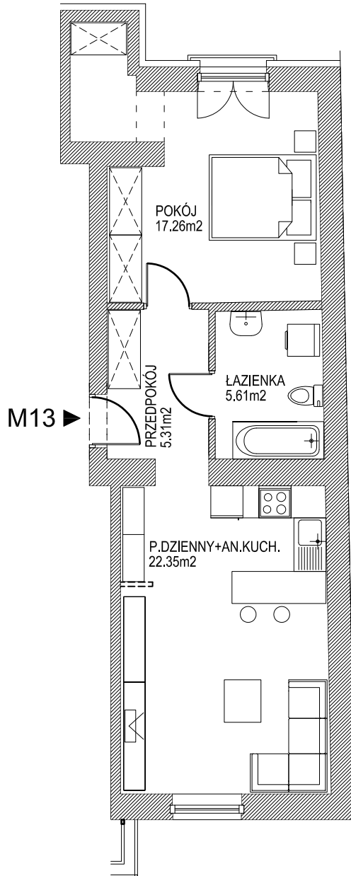
SCHEMAT MIESZKAŃ W KONDYGNACJI 4 PIĘTRA
